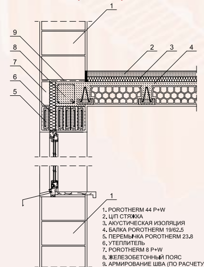
Сборная перемычка
