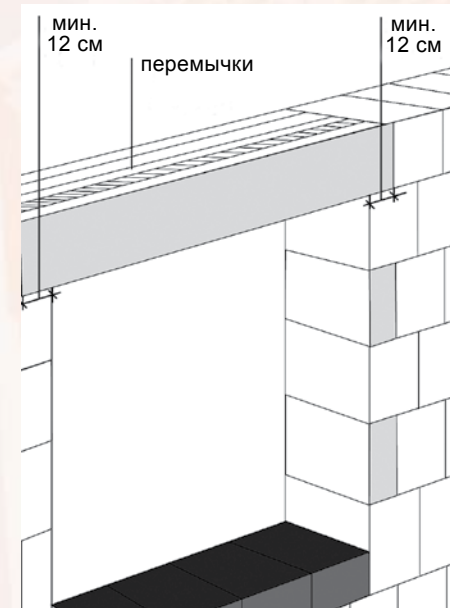
Сборная перемычка
