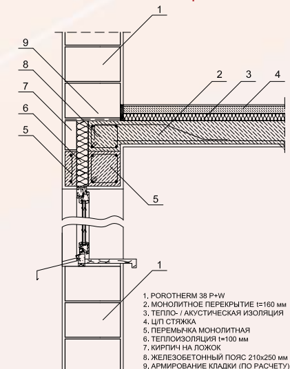
Монолитная перемычка
